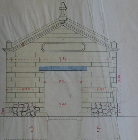
Play au-dessus des fondations
