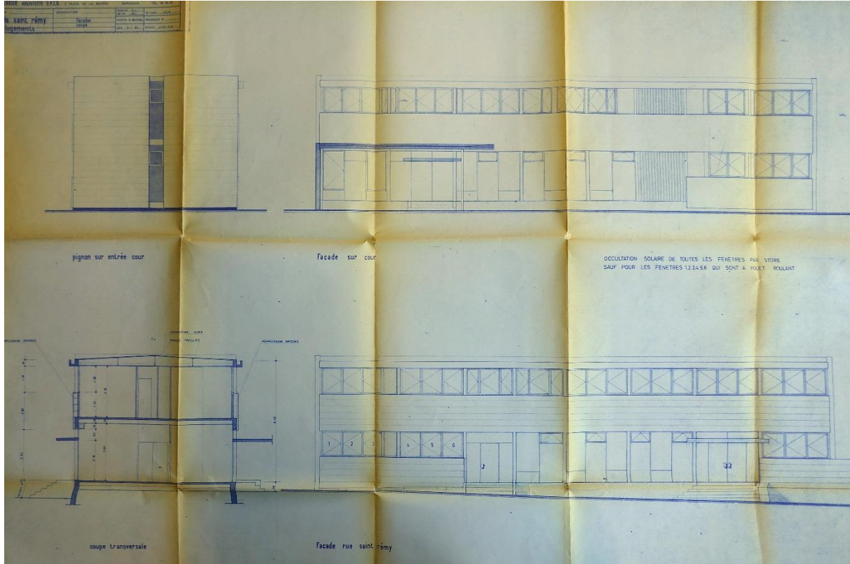
Élévation du bâtiment rue Saint-Rémi par Francisque Perrier, 1962 (ABM, Bordeaux, 6910 M 7)
