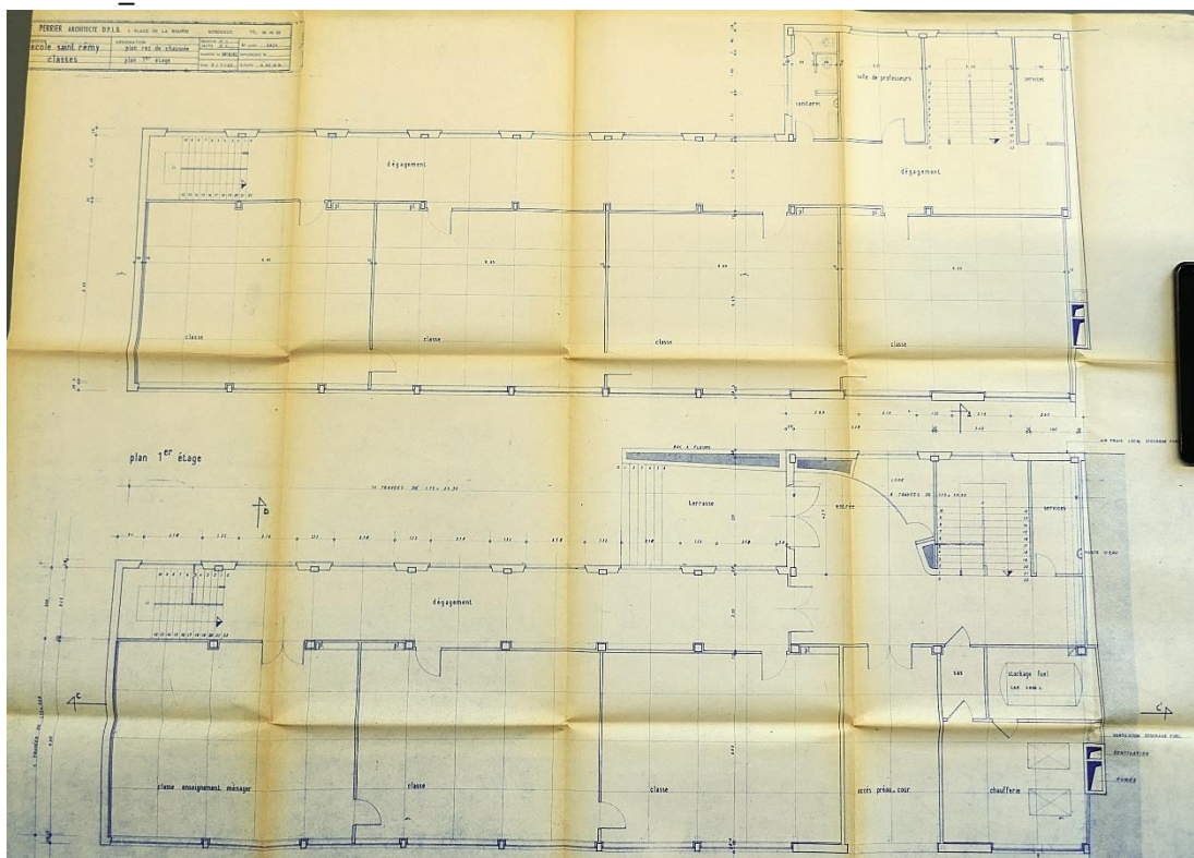
Plan (rdc et étages) du bâtiment rue du Pont-de-la-Mousque par Francisque Perrier, 1962 (ABM, Bordeaux, 6910 M 7)
