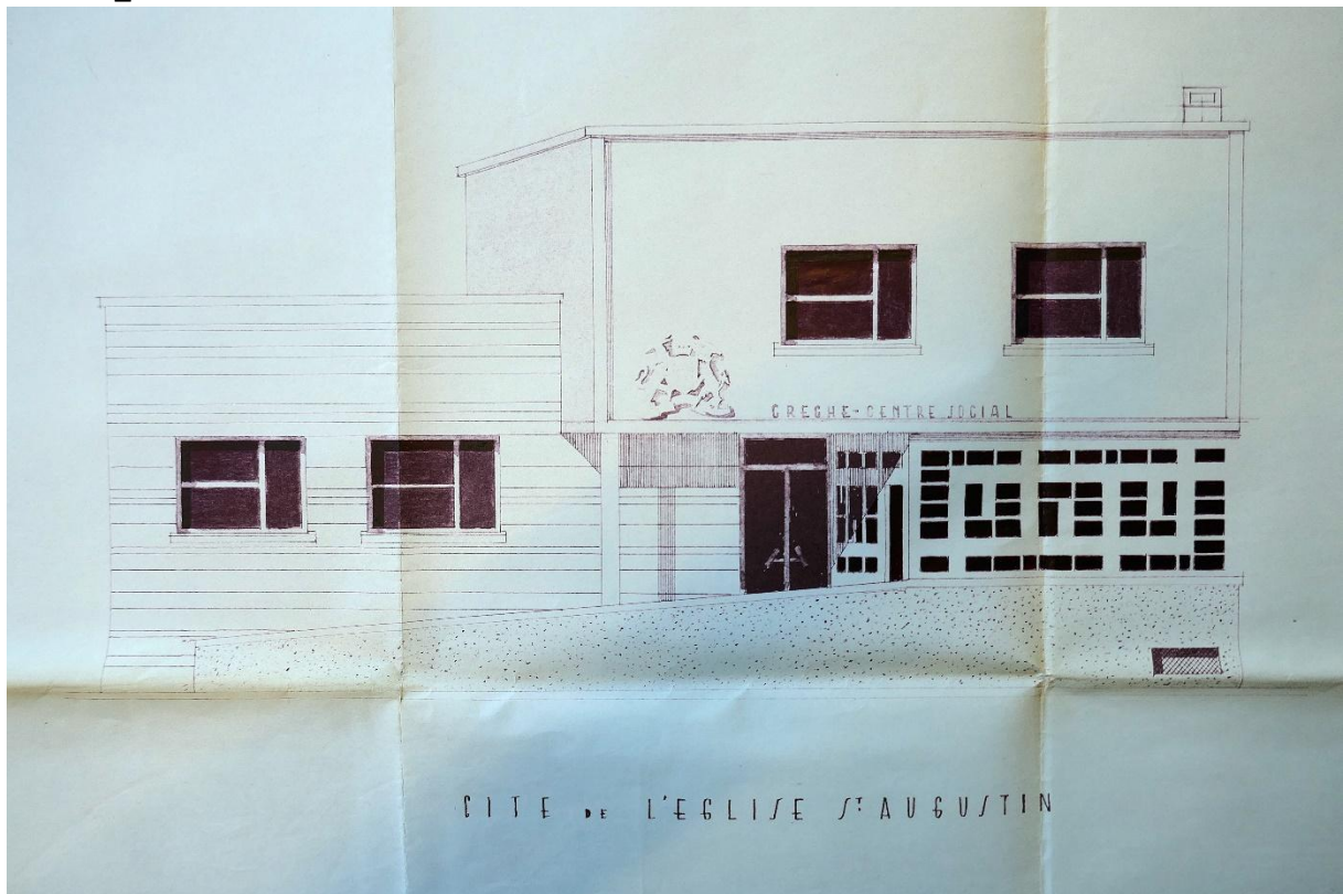
Élévation de la façade nord, mêlant les matériaux traditionnels et modernes, par l'architecte A. Thierry, 1960 (ABM, Bordeaux, 14 W 8552)
