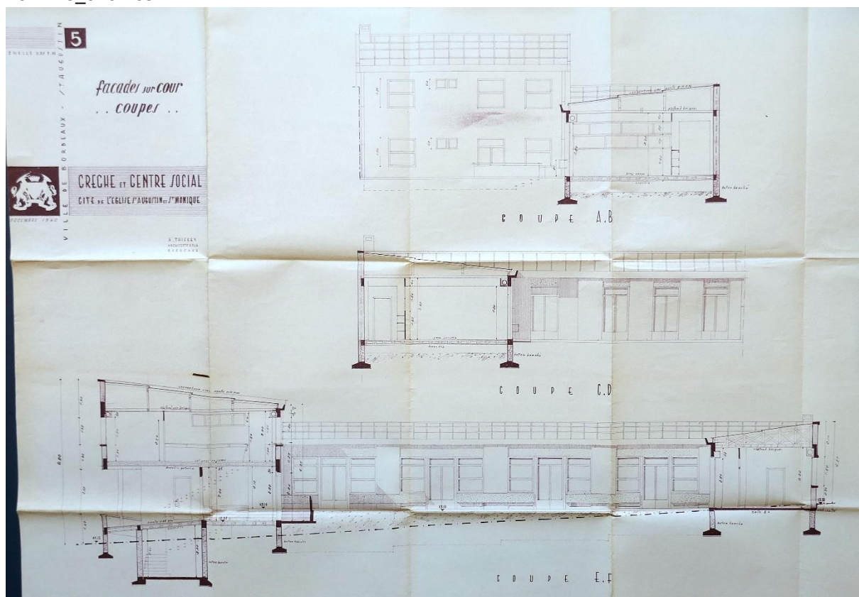
Coupe des bâtiments de la crèche par l'architecte A. Thierry, 1960 (ABM, Bordeaux, 14 W 8552)
